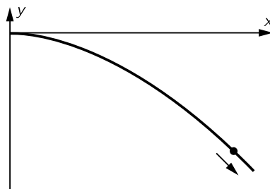
图 8.3: 物体二维运动的描述和它的速度的计算
