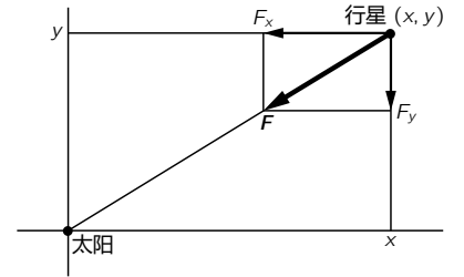
图 9.5: 作用在行星上的太阳引力
